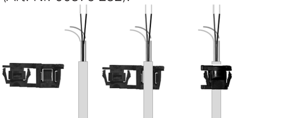
Vorgehensweise bei normalem Installationskabel
