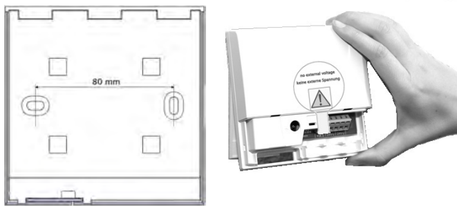
Wandmontageplatte
