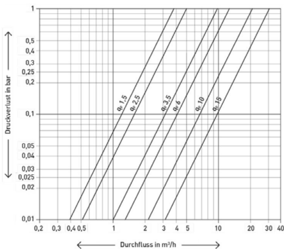
Druckverlustkurve
