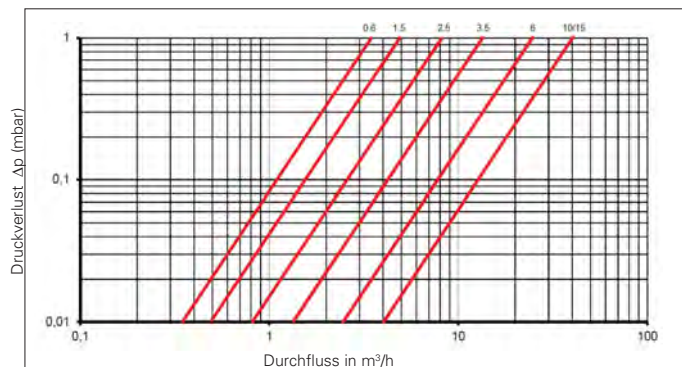
Druckverlustkurve
